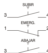
Botonera Subir - Emergencia - Abajar S-Q3A
